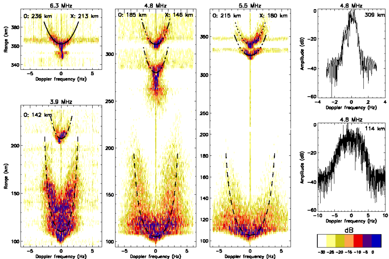
Figure 7 : Spectre de l'intensité du Doppler en fonction de l'altitude. La forme en U est typique des réflexions obliques en région E et région F. Deux exemples de puissance spectrale du Doppler en région E, à 114 km et en région F à 309 km
